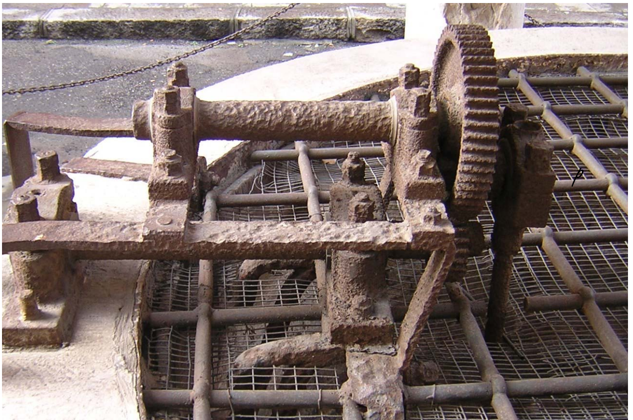
Particolare del sistema di sollevamento in uso presso la cisterna di P.za Sarzano (foto G. Temporelli)
